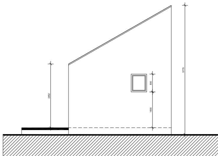
POHĽAD VÝCHODNÝ
