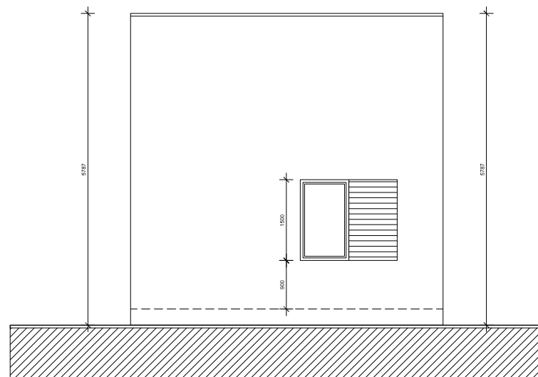
POHĽAD SEVERNÝ
