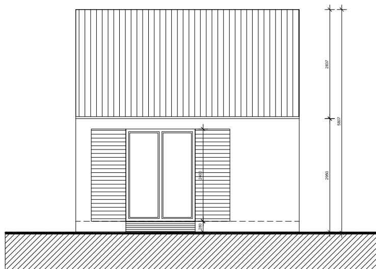
POHĽAD JUŽNÝ
